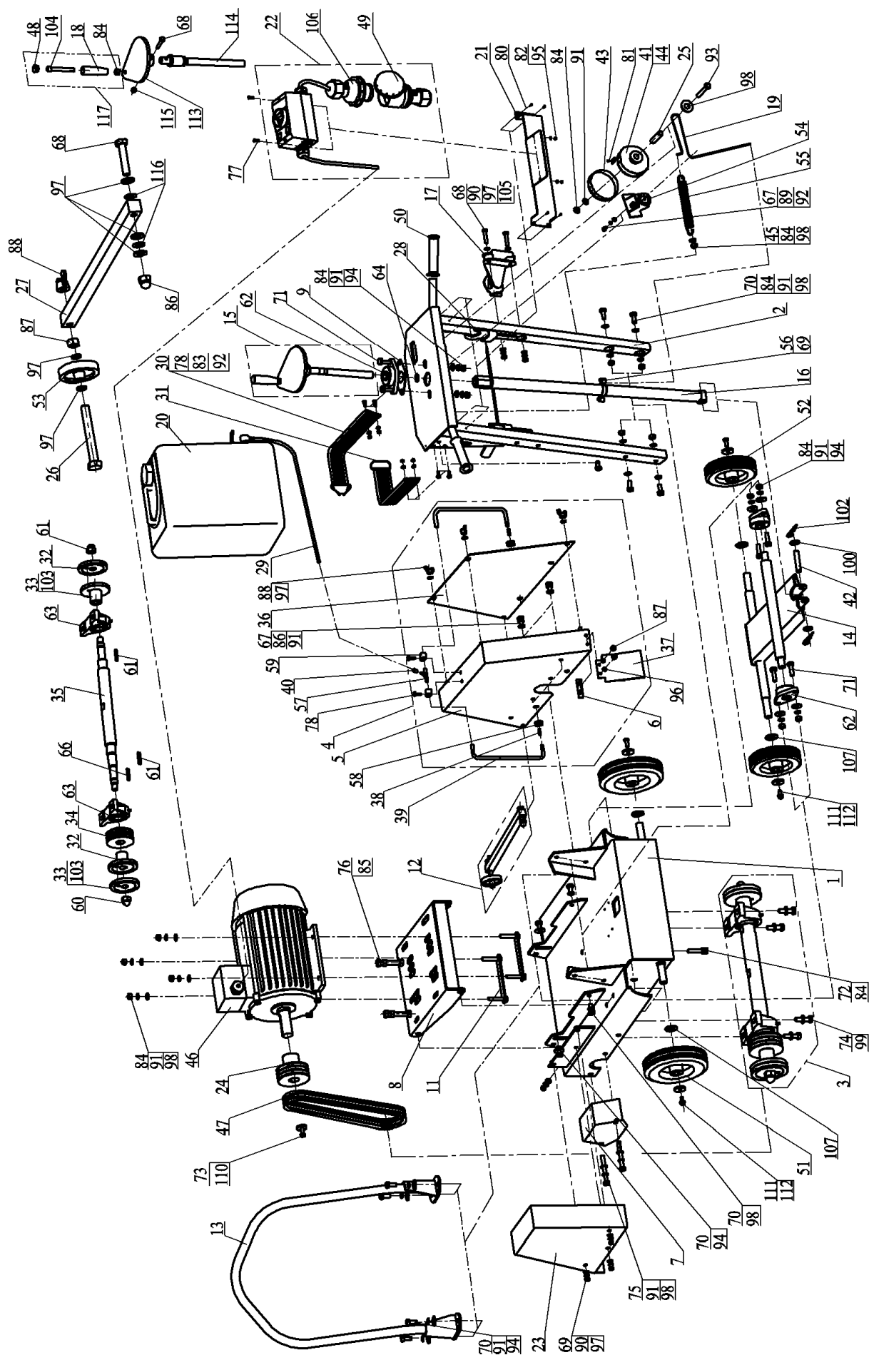
Рисунок 17 – Компоновка резчика
