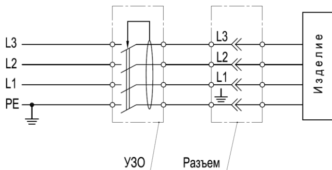
Рисунок 7 - Схема подключения УЗО
